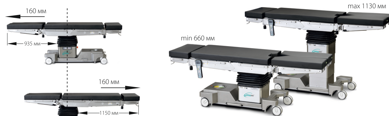
Широкий диапазон регулирования высоты панели
