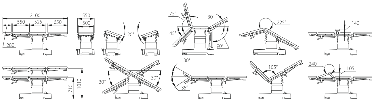
Механический излом спинной секции (опция)
